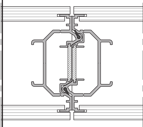
Detail onderlinge aansluiting tussen 2 panelen
